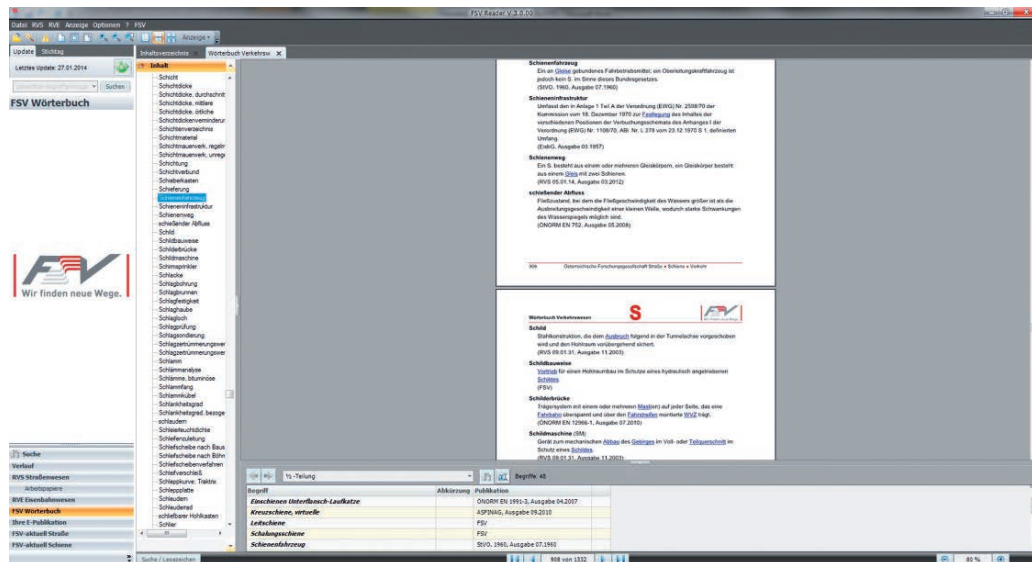
BILD 2: Digitale Suchansicht
